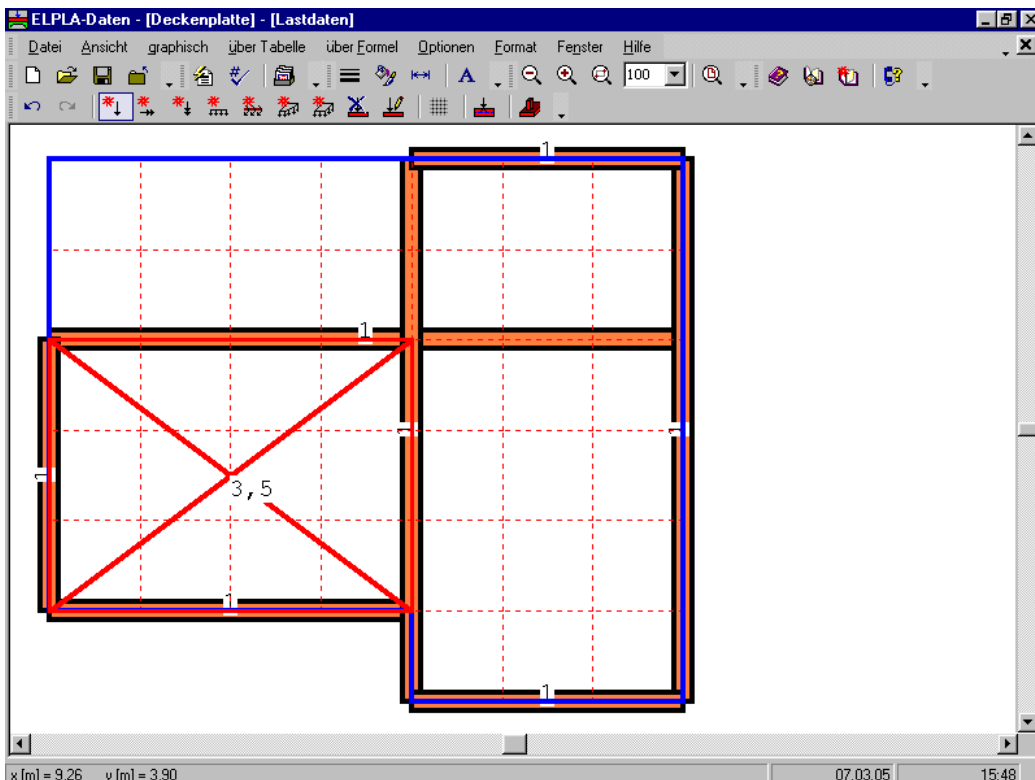
Bild 2-34 Die erste Flächenlast P = 3.5 [kN/m 2 ] auf dem Bildschirm
