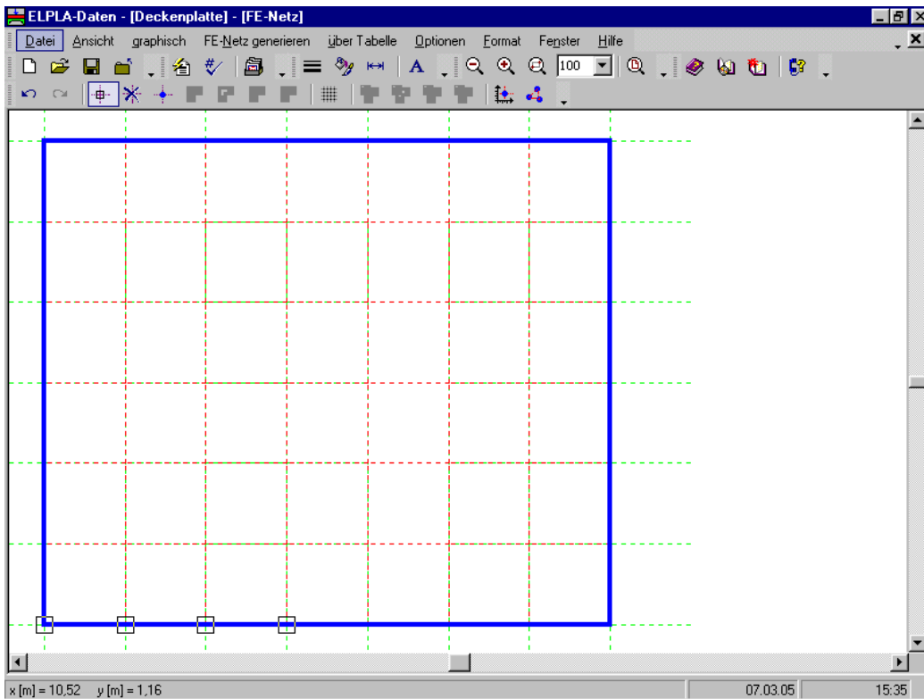
Bild 2-12 Generiertes FE-Netz nach dem Markieren der unnötigen 4 Knoten (unten links)
