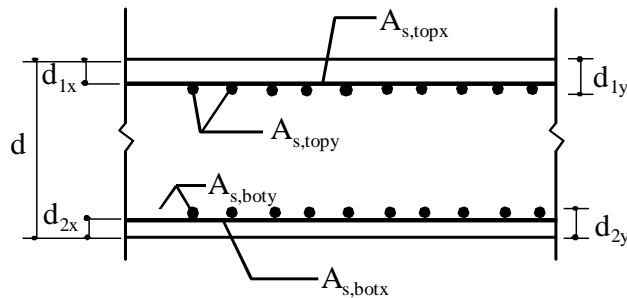
Bild 2-30 Schnittgeometrie und Bewehrung parallel zur x -Richtung
