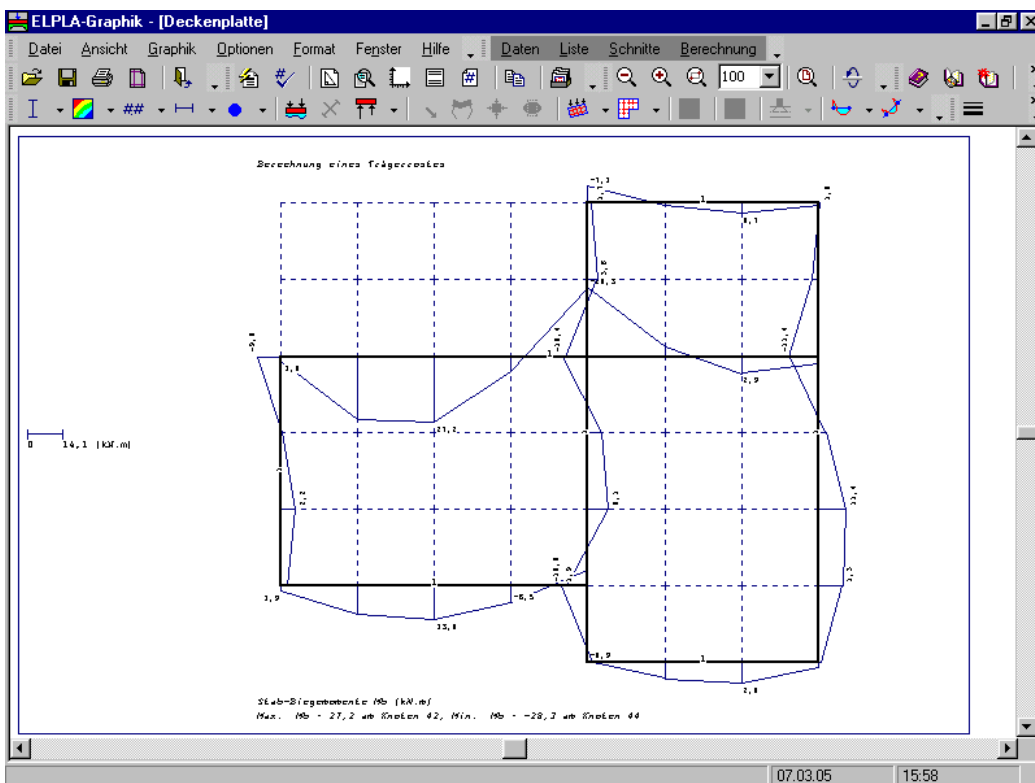
Bild 2-41 Stab-Biegemomente M_b
