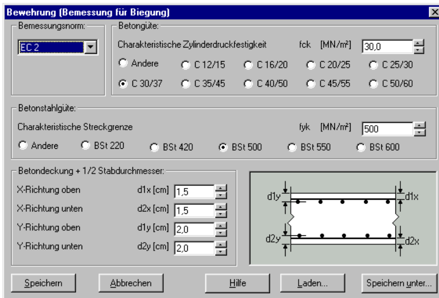
Bild 2-31 Dialogfeld "Bewehrung"
