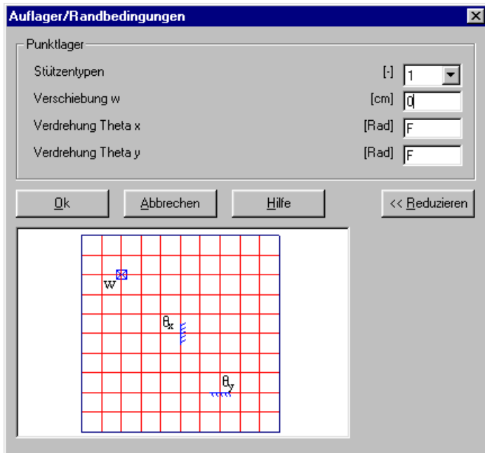
Bild 2-25 Dialogfeld "Auflager/ Randbedingungen"
