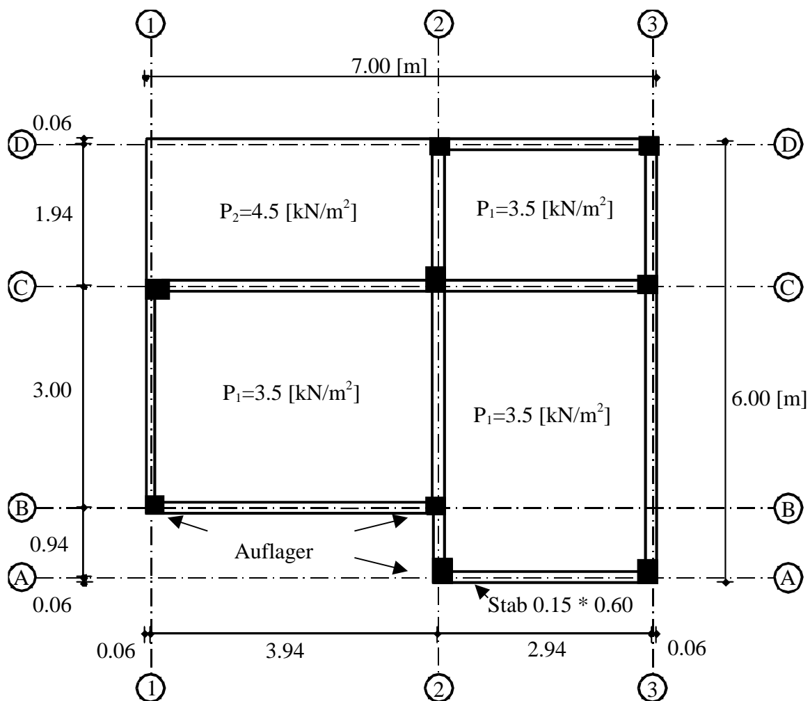
Bild 2-1 Deckenplatte mit Flächenlasten P_1 und P_2 , mit Stäben und 9 Auflagern
