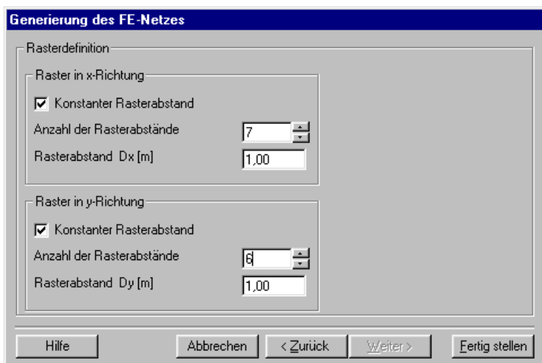
Bild 2-10 Dialogfeld "Rasterdefinition"
