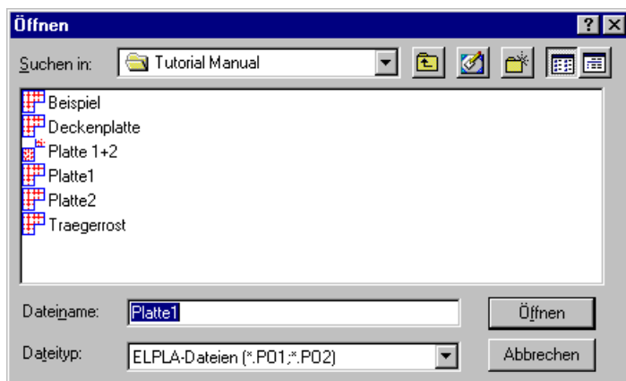
Bild 3-33 Dialogfeld "Öffnen"
