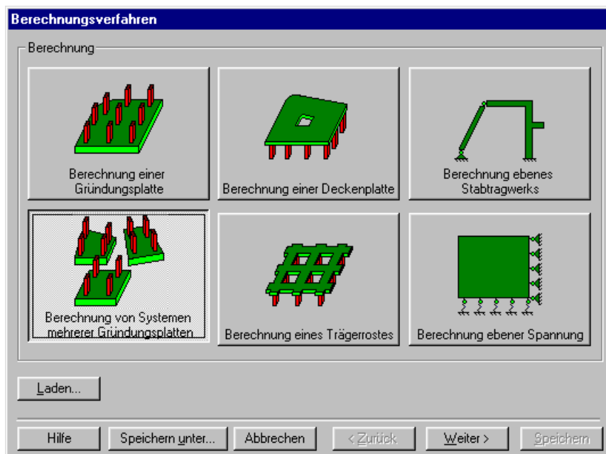
Bild 3-31 Optionsfeld "Berechnung"
