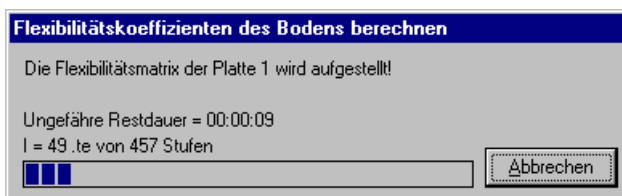
Bild 3-39 Berechnungsfortschrittsmenü
