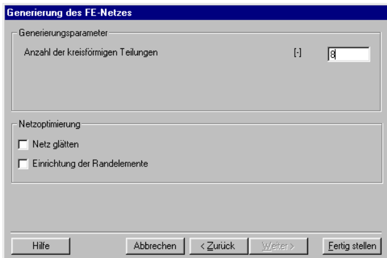
Bild 3-11 Dialogfeld "Generierungsparameter"
