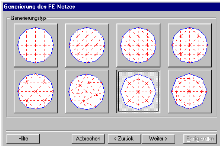
Bild 3-10 Menü "Generierungstyp"
