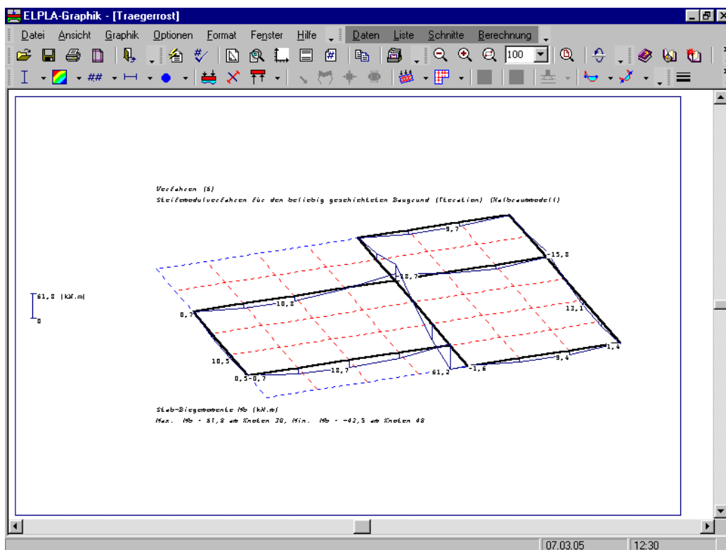
Bild 4-32 Stab-Biegemomente M_b
