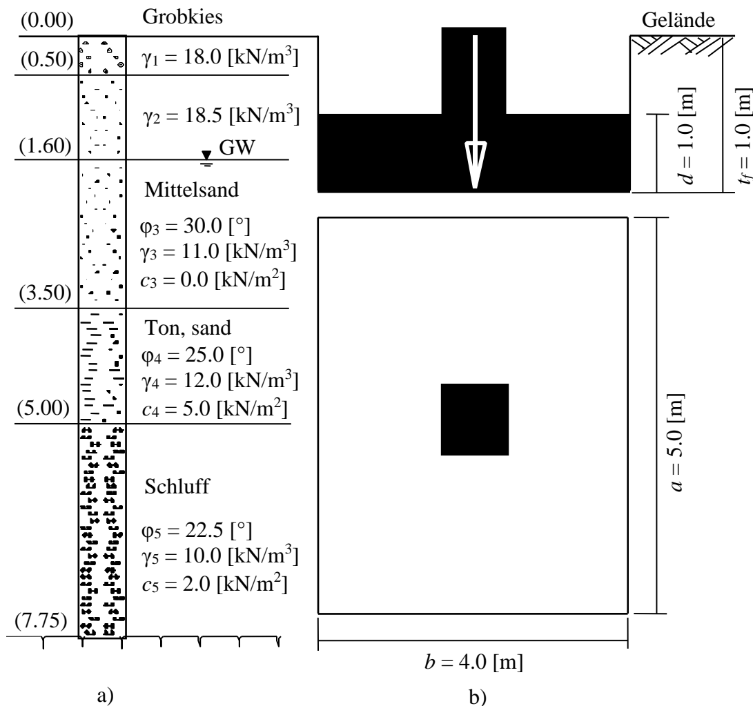
Bild 15 a) Querschnitt durch den Baugrund unter dem Fundament b) Grundriss des Fundaments mit Abmessungen
