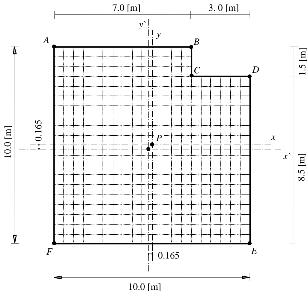
Bild 17 Abmessungen der Platte und FE-Netz
